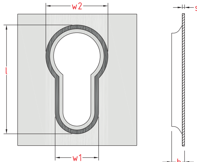
Otvor: Konfekcijsko saće
