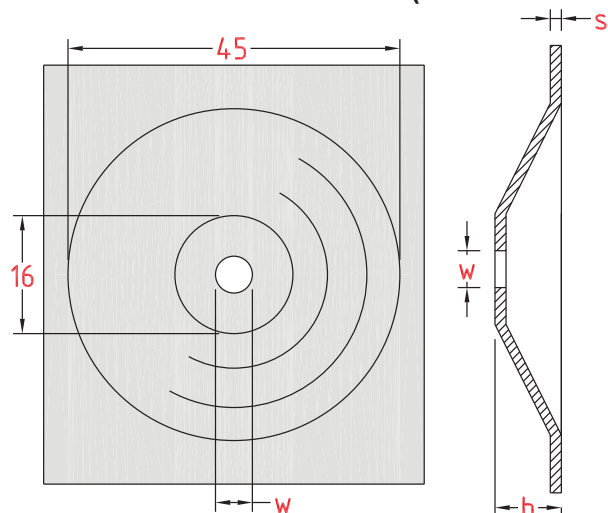
Otvor: Distancer DR 45 - 16 (konusni izvučeni)
