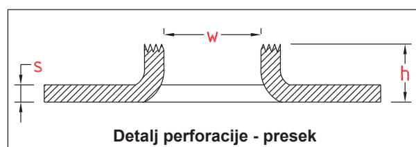
Okrugli cepani otvor
