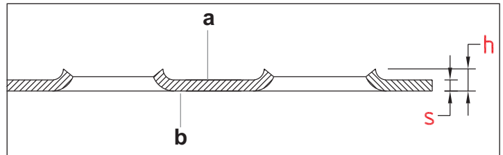
DETALJ PERFORACIJE - PRESEK
