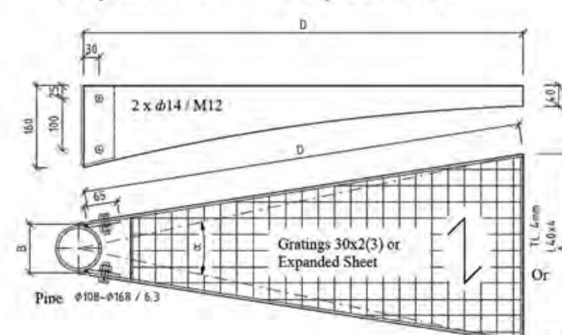
Spiralni rešetkasti stepenik / Спиральный шаг решетка
