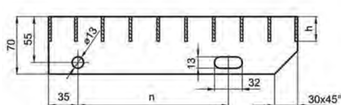
Stepenik – model RS (sa punim flahom): bez protivkliznog nagaznog profila / Решетчатый шаг модель RS
