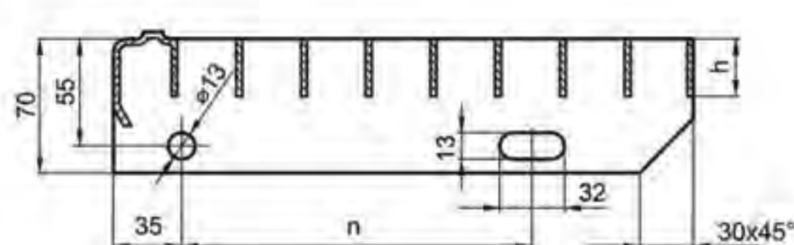
Stepenik – modeli RSP (sa poluflahom) sa protivkliznim nagaznim profilom / Шаг решетки модель RSP
