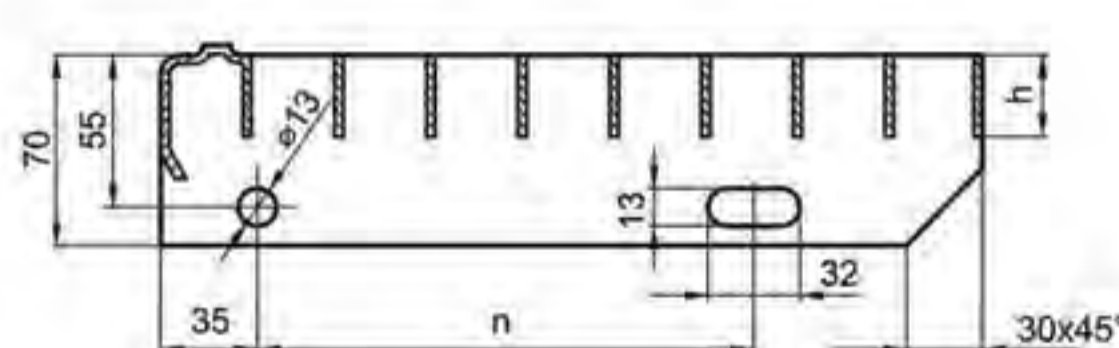
Stepenik – modeli RSP (sa poluflahom) sa protivkliznim nagaznim profilom Stair step - model RSP
