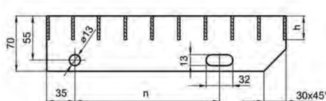
Stepenik – model RS (sa punim flahom): bez protivkliznog nagaznog profila: Stair step - model RS
